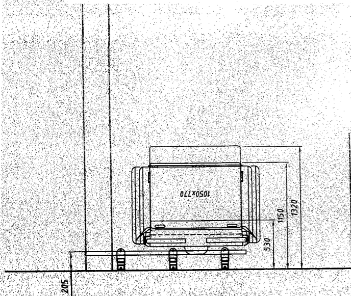
Šikmá plošina 1 np vstup přímá levá zdvih 300 mm
