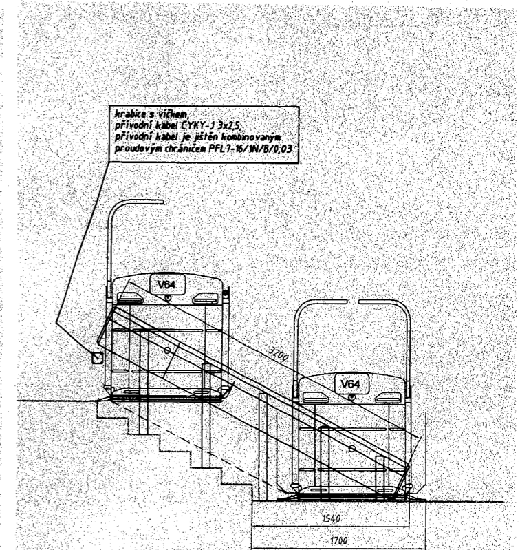
Šikmá plošina 3 np chodba přímá pravá zdvih 920 mm
