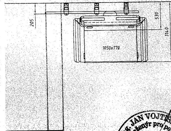
Šikmá plošina 1 np chodba přímá pravá zdvih 300 mm
