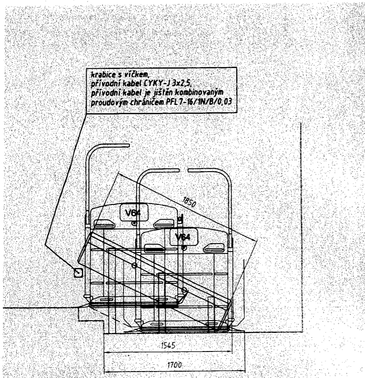
Šikmá plošina 1 np vstup přímá levá zdvih 300 mm
