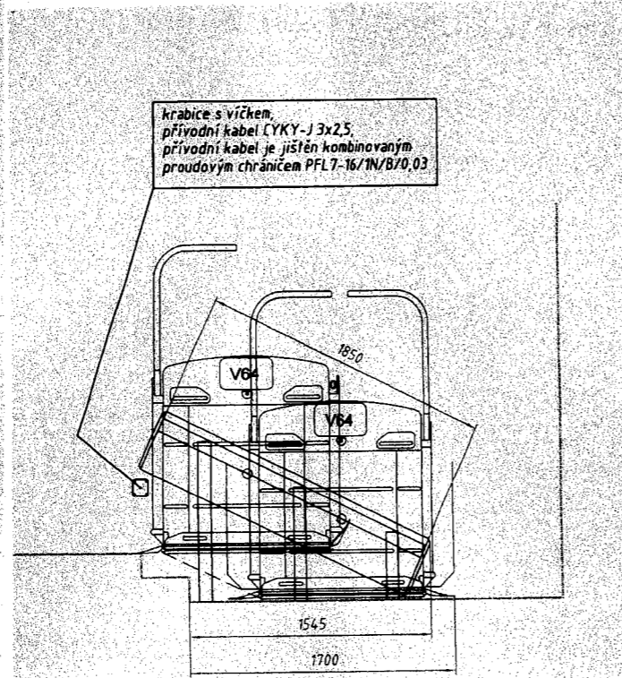
Šikmá plošina 1 np chodba přímá pravá zdvih 300 mm
