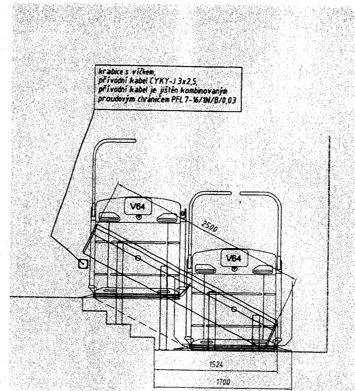
Šikmá plošina 2 np chodba přímá pravá zdvih 600 mm
