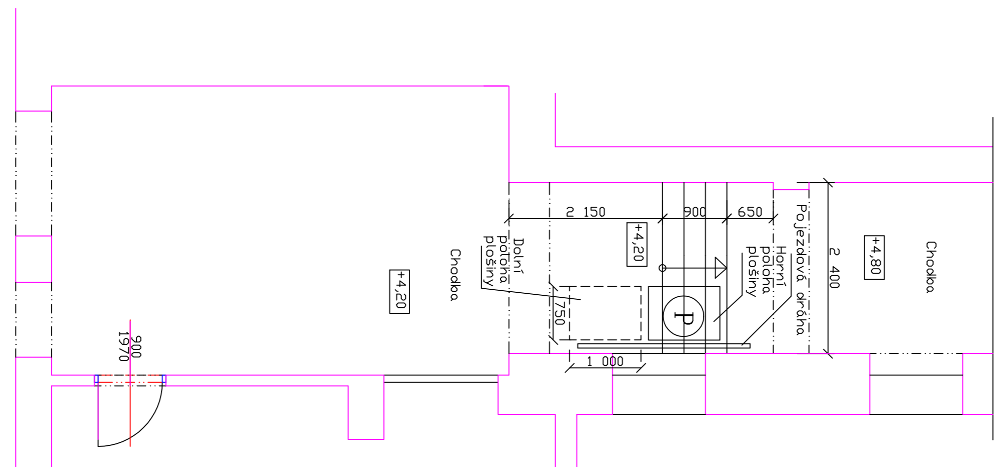
Púdorys schodiště
