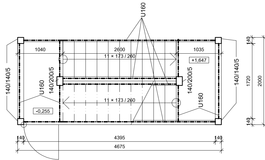
PŮDORYS
