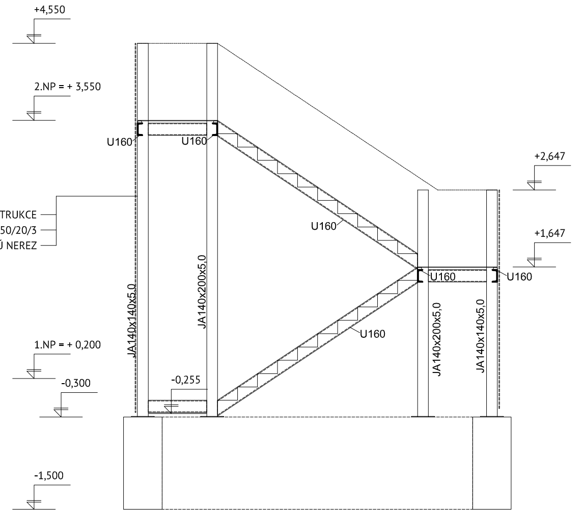
SVISLÝ ŘEZ
