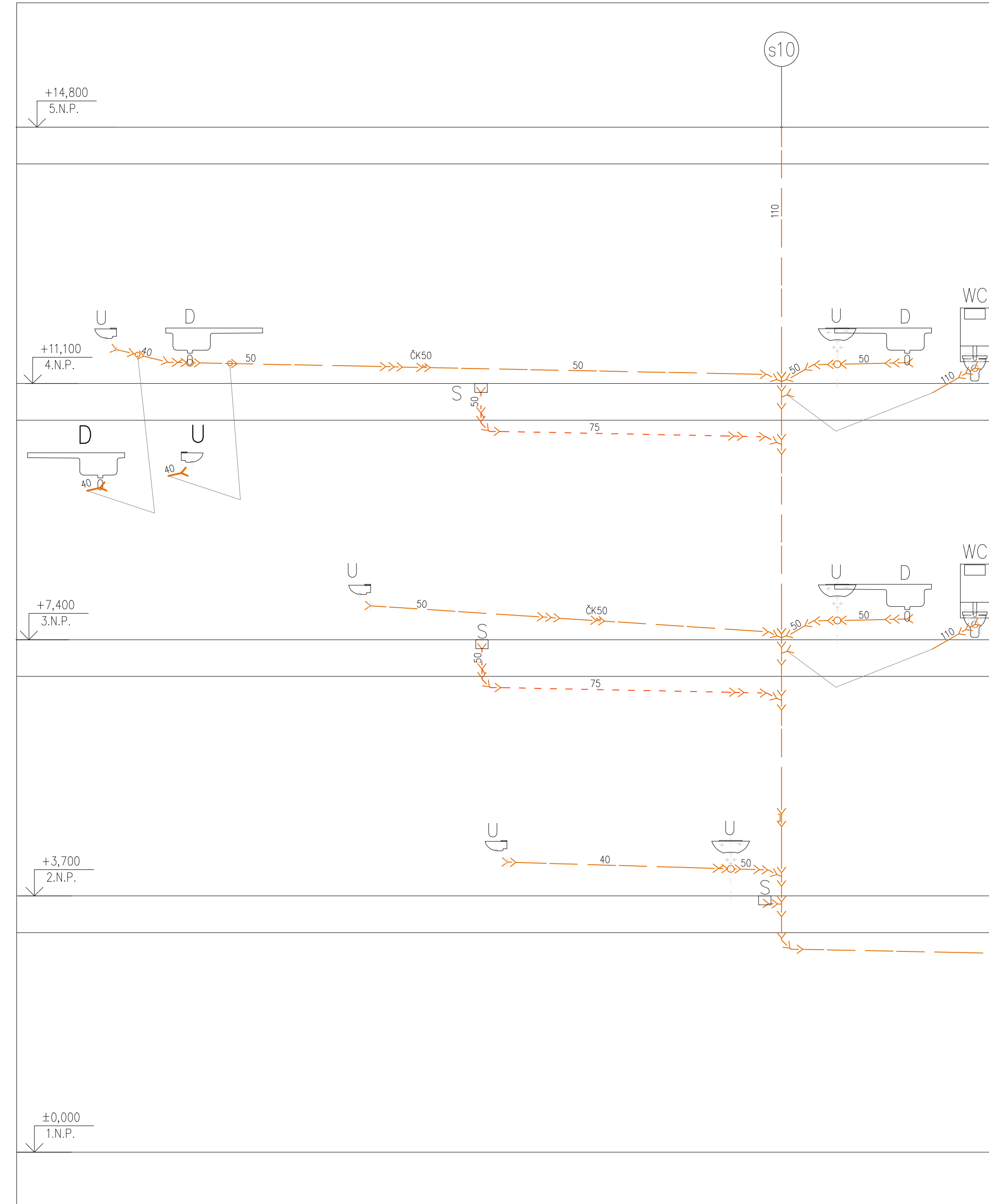
řez (stoupačka) s10
