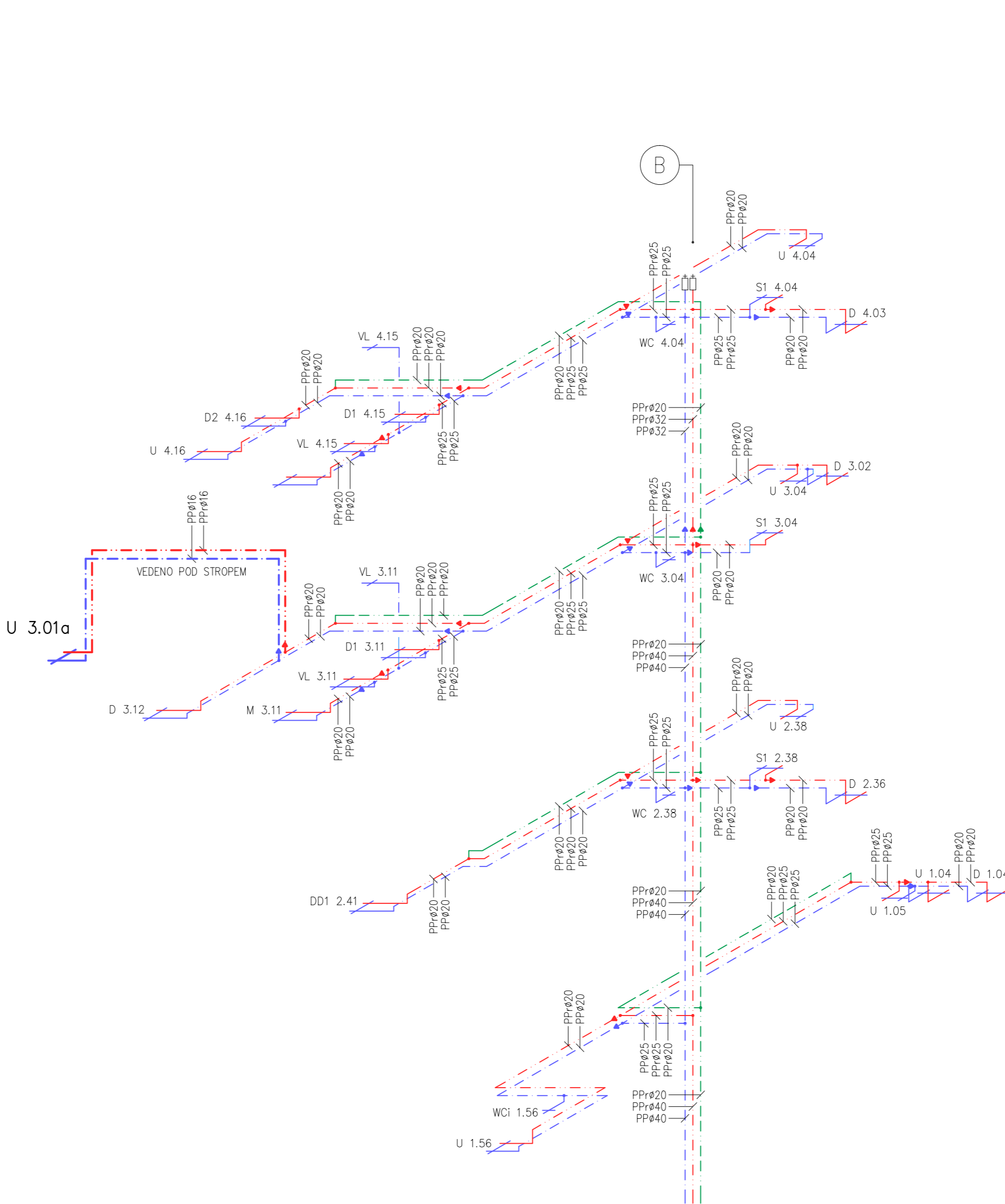
axonomie vodovodu
