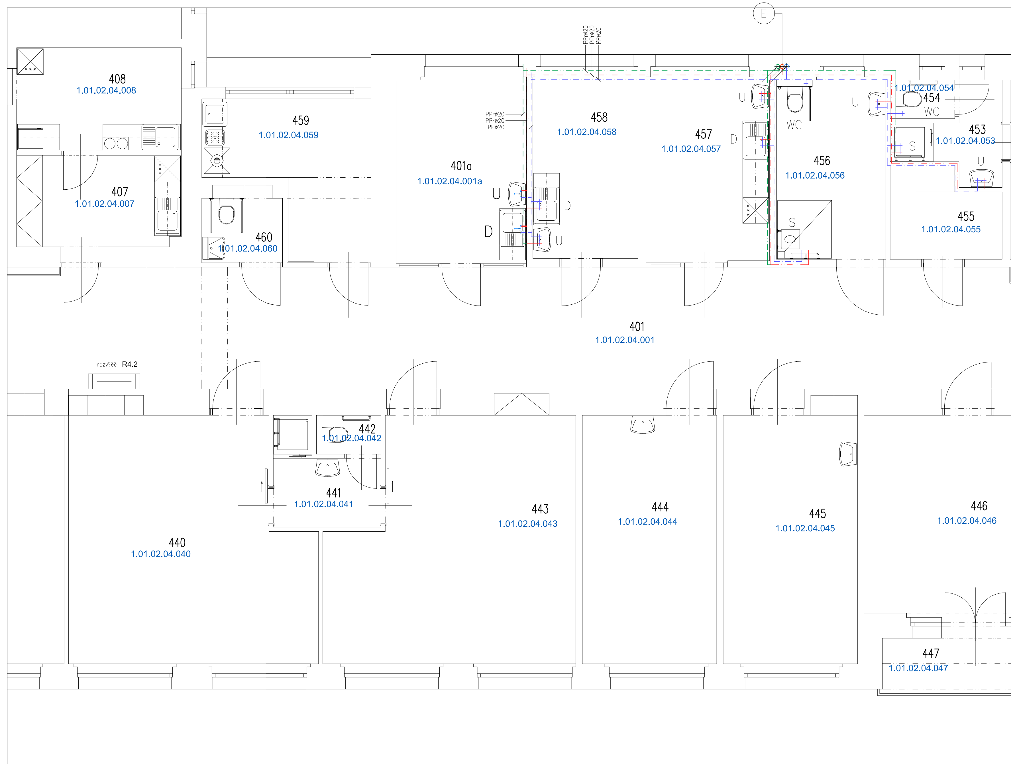
PŮDORYS 4.N.P. M 1 : 50
