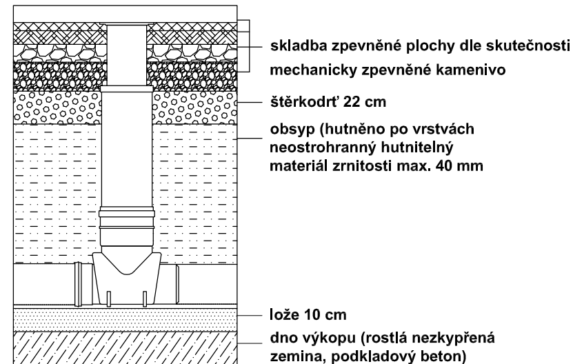
VZOROVÝ ŘEZ KANALIZAČNÍ ŠACHTY BEZ MĚŘÍTKA
