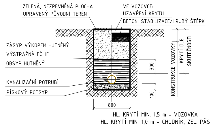
VZOROVÝ PŘÍČNÝ ŘEZ VÝKOPEM ULOŽENÍ KANALIZAČNÍHO POTRUBÍ - BEZ MĚŘÍTKA
