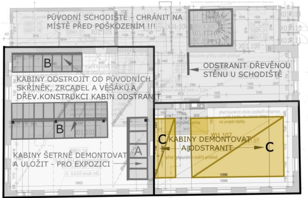
Umístění 23 ks převlékacích kabin cca z roku 1970 v prostoru šaten - označeny žlutě
