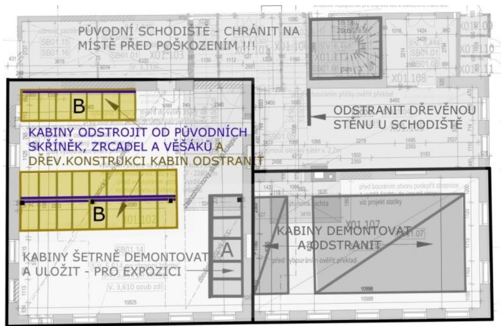
Umístění 25 ks převlékacích kabin cca z roku 1950 v prostoru odpočívárny - označeny žlutě, modrá barva upozorňuje na původní mobiliář uvnitř kabin (poličky, zrcadla, háčky aj.), které budou šetrně demontovány a uloženy.
